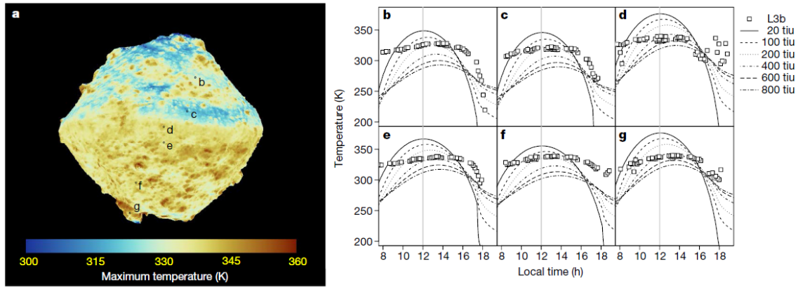
図 1：左の図は小惑星リュウグウの 1 日の最高温度の分布。右のグラフは、各地点で観測された一日の温度変化（□マーク）と理論計算に基づく予測値（実線と破線）の比較。理論計算では一様な熱慣性を仮定し熱慣性の値を変化させて計算している。
