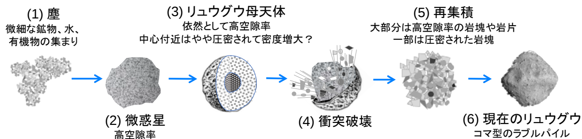
図2：リュウグウ形成のシナリオ ©Okada et al., Nature 2020
