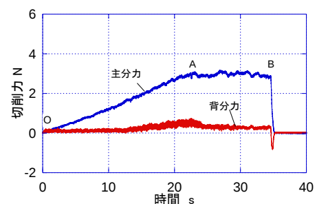
図2 切削力変化
