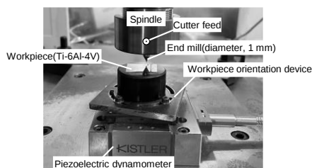
図 3 エンドミル切削試験
